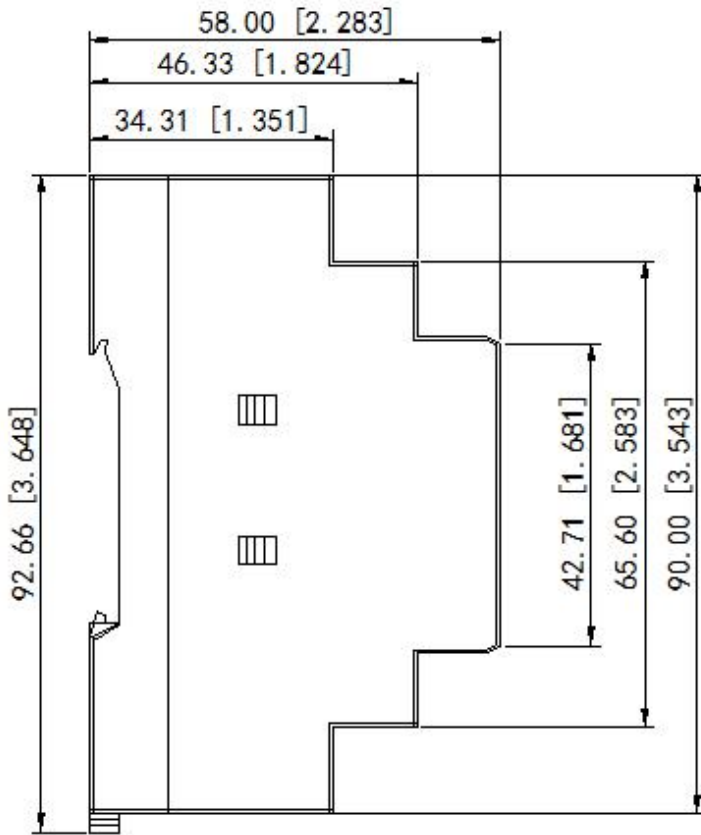
左视图 Leftview
