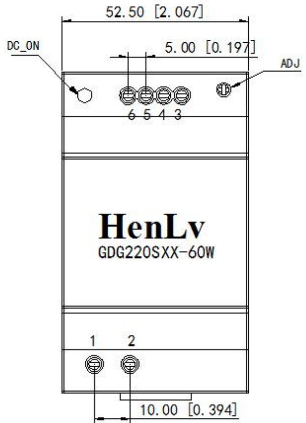
前视图 Frontview
